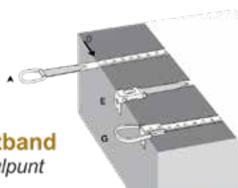
Stalen meetband Bandeindes en nulpunt
